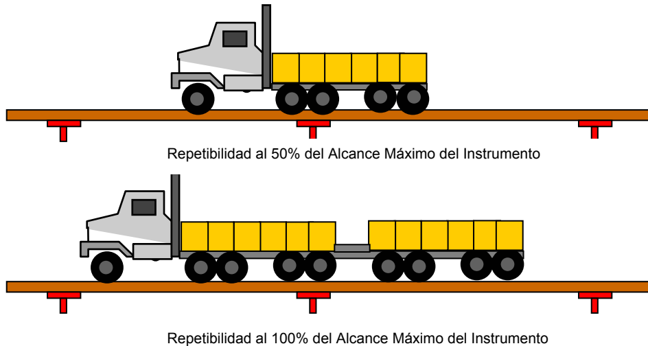
figura 4.- Prueba de Repetibilidad.
