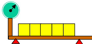
figura 6.- Plataforma con 20% del Max. en masas patrón
