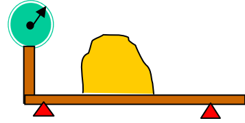
figura 7.- Plataforma con masa de sustitución por el 20% del Max.
